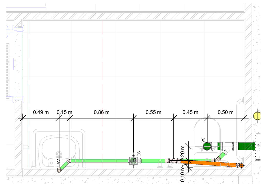
3 Detalhe 2 1 : 25
