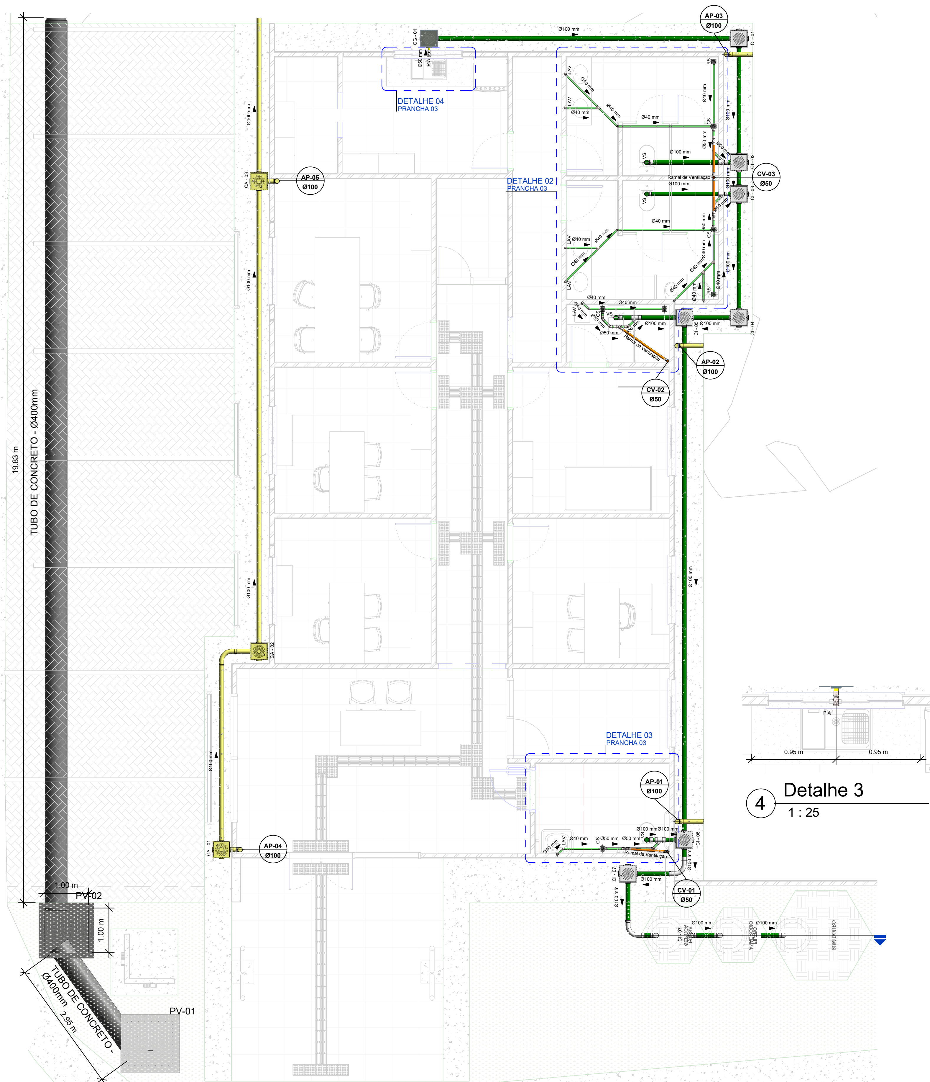
1 Térreo-ESG 1 : 50
