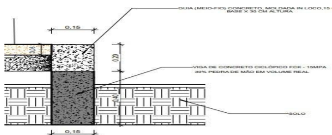
Imagem Capturada: Projeto Arquitetônico prancha 01/0
