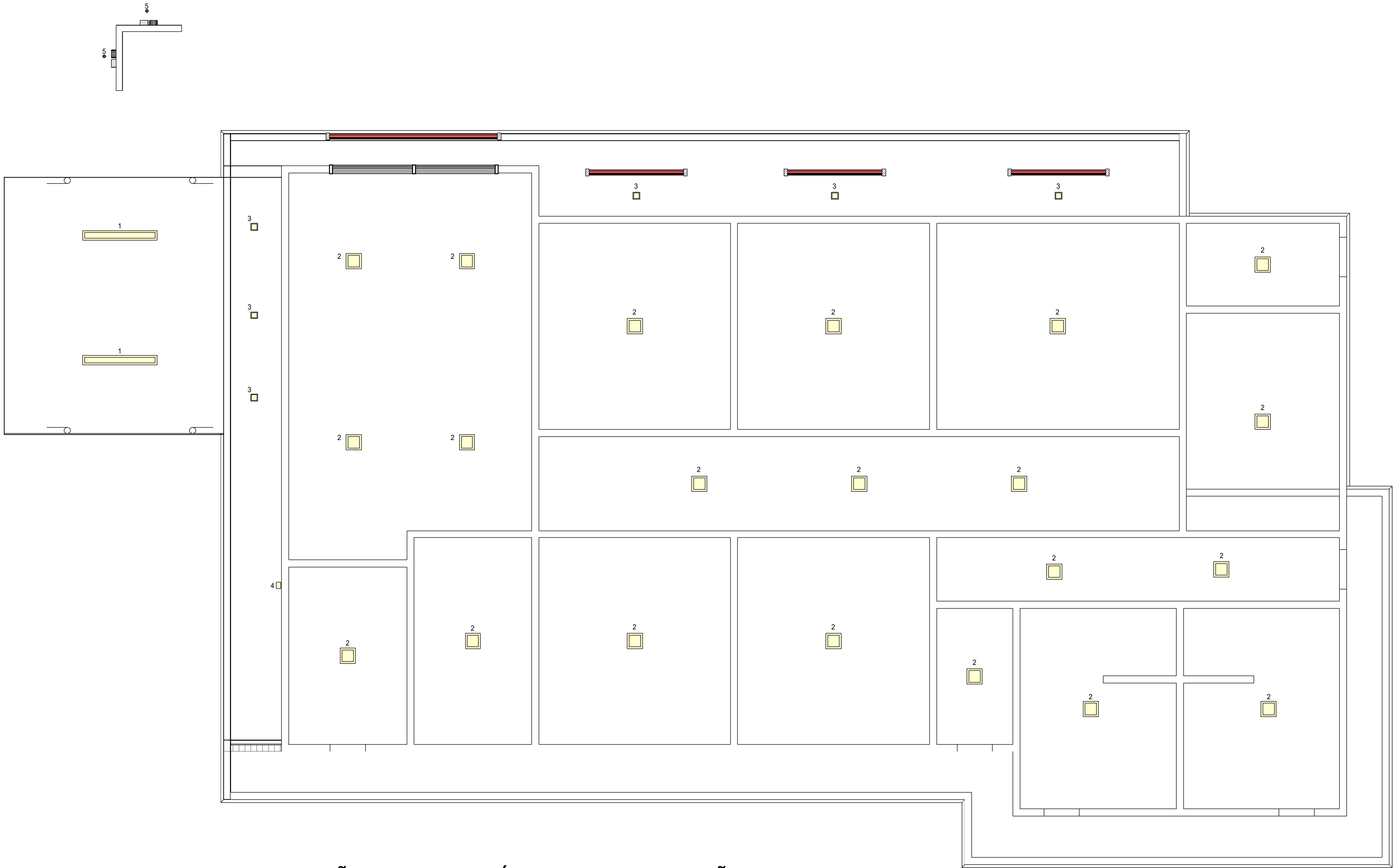
1 PLANTA BAIXA - LOCAÇÃO DE LUMINÁRIAS E PAGINAÇÃO DE FORRO 1 : 50
