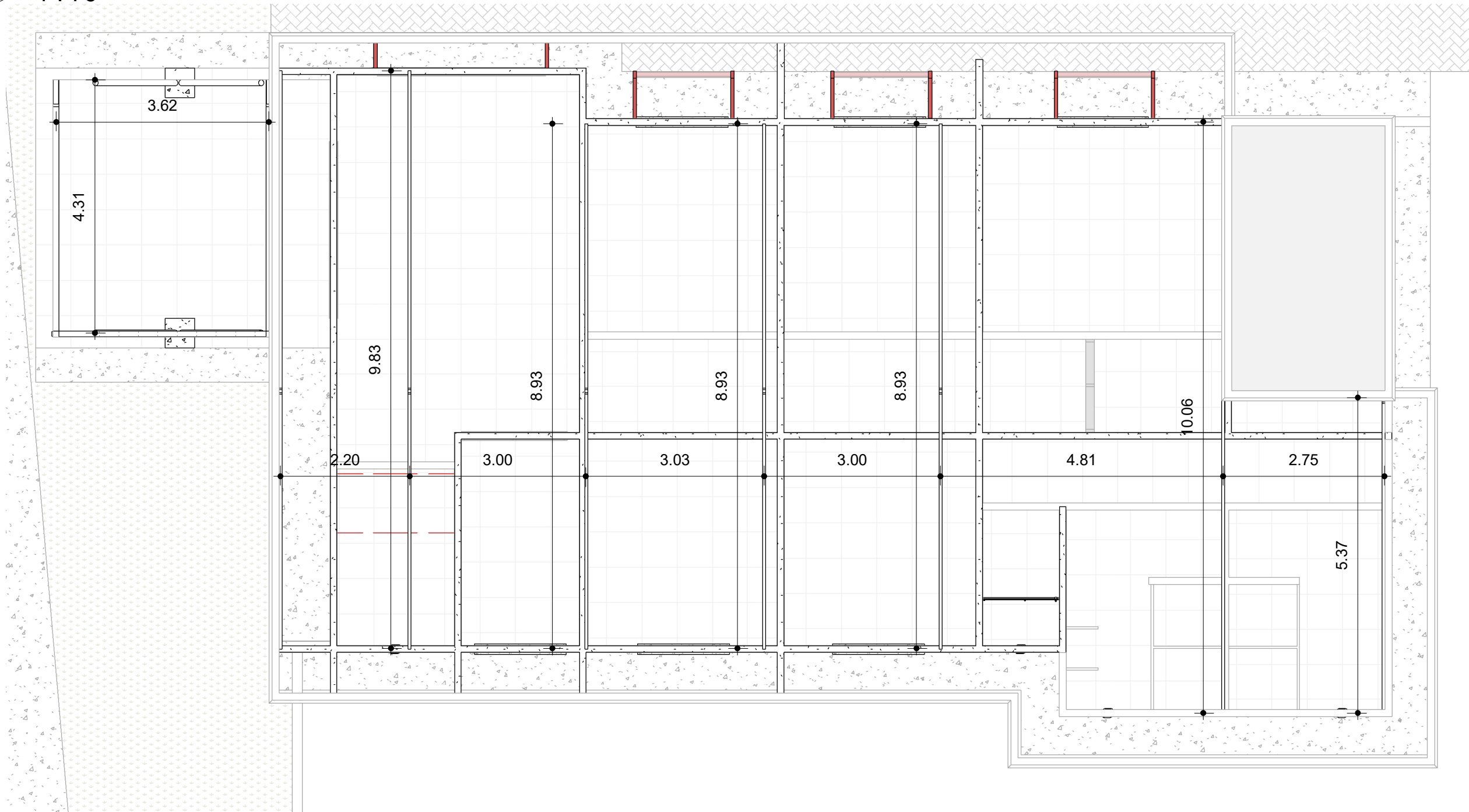
1 PLANTA DE COBERTURA 1 : 75
