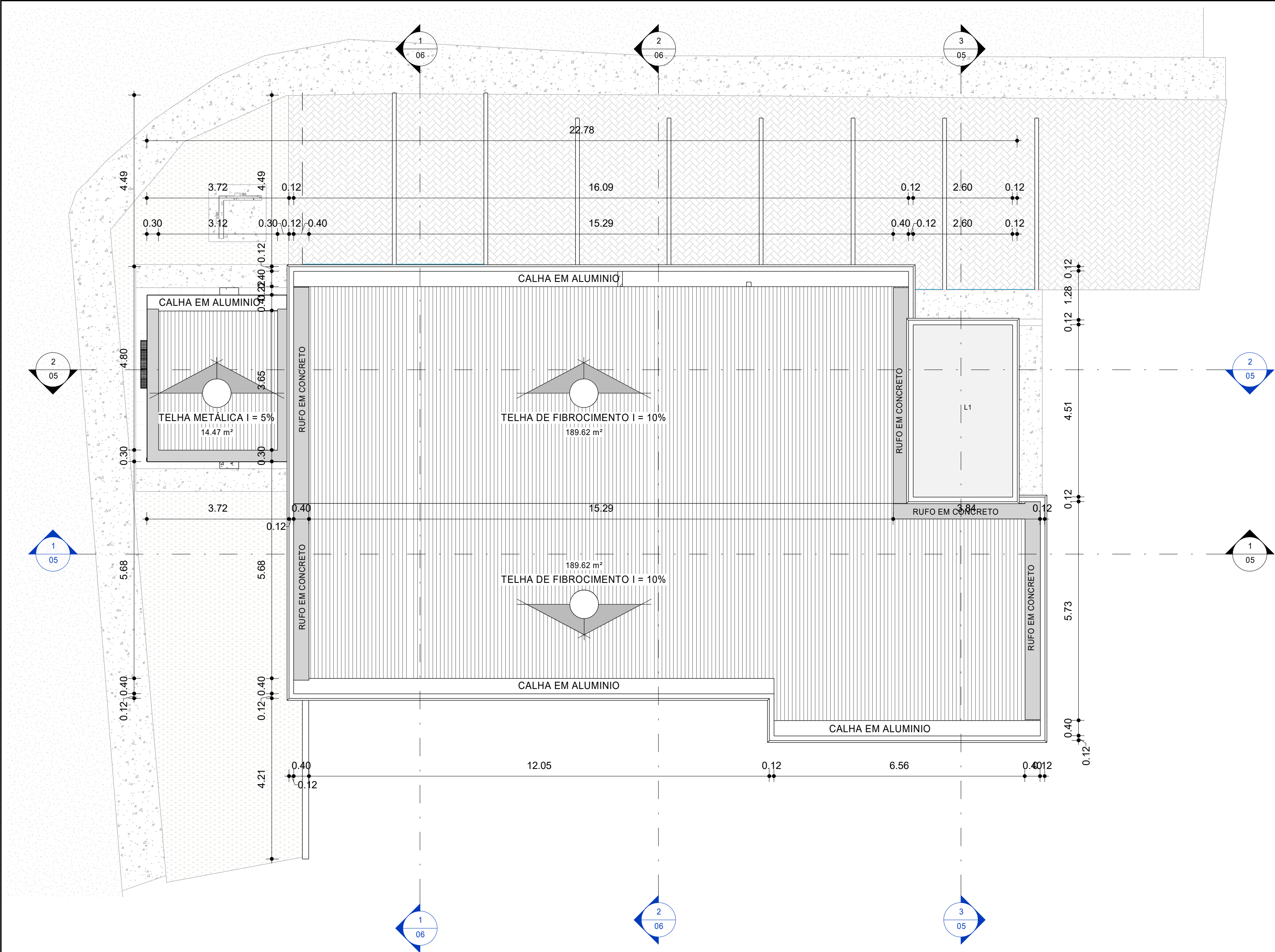
1 PLANTA DE COBERTURA 1 : 75
