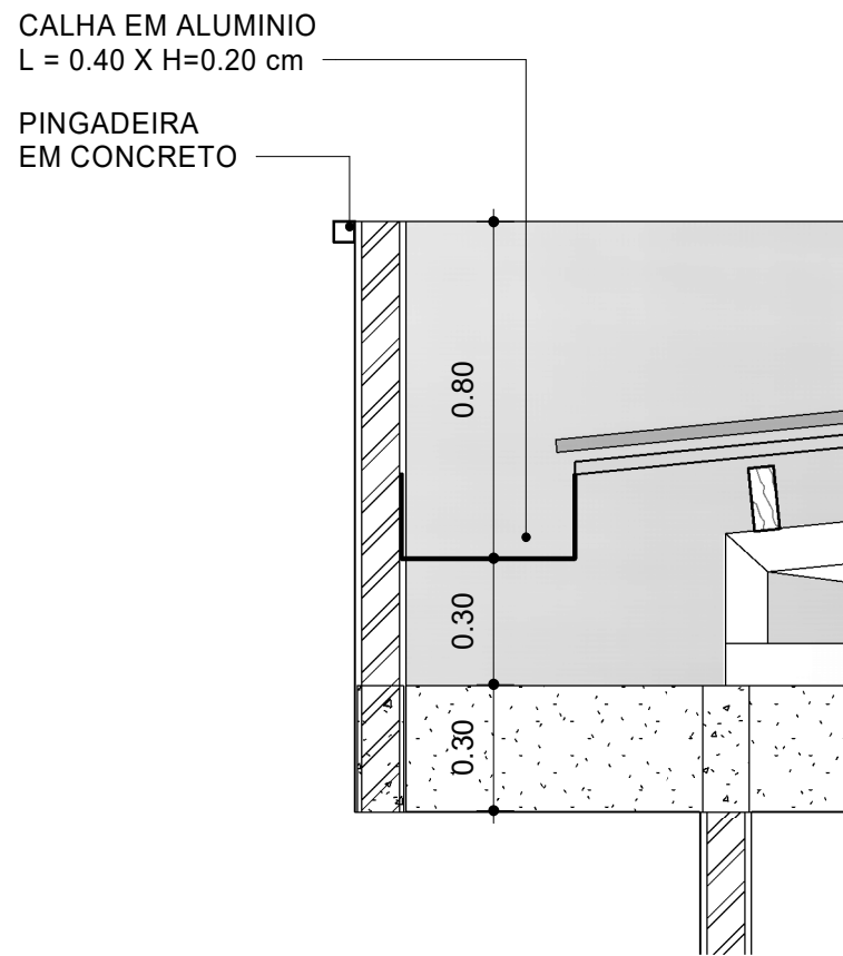
3 DET. CORTE CALHA DE ALUMINIO 1 : 20
