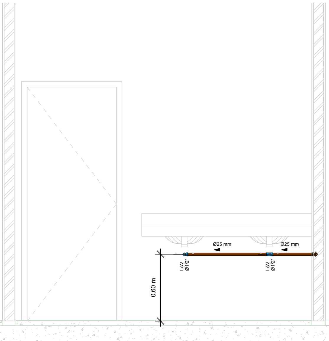
4 Elevação 06 1 : 20
