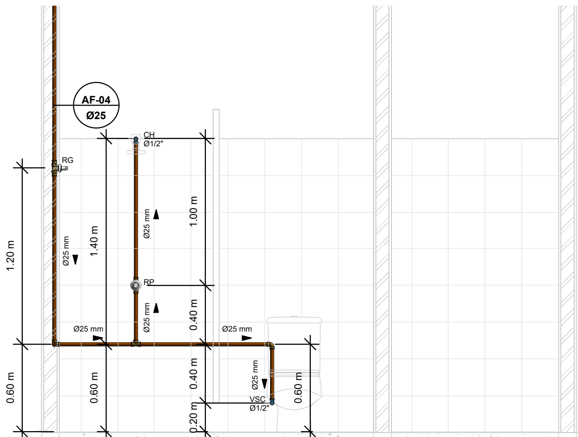
7 Elevação 05 1 : 25
