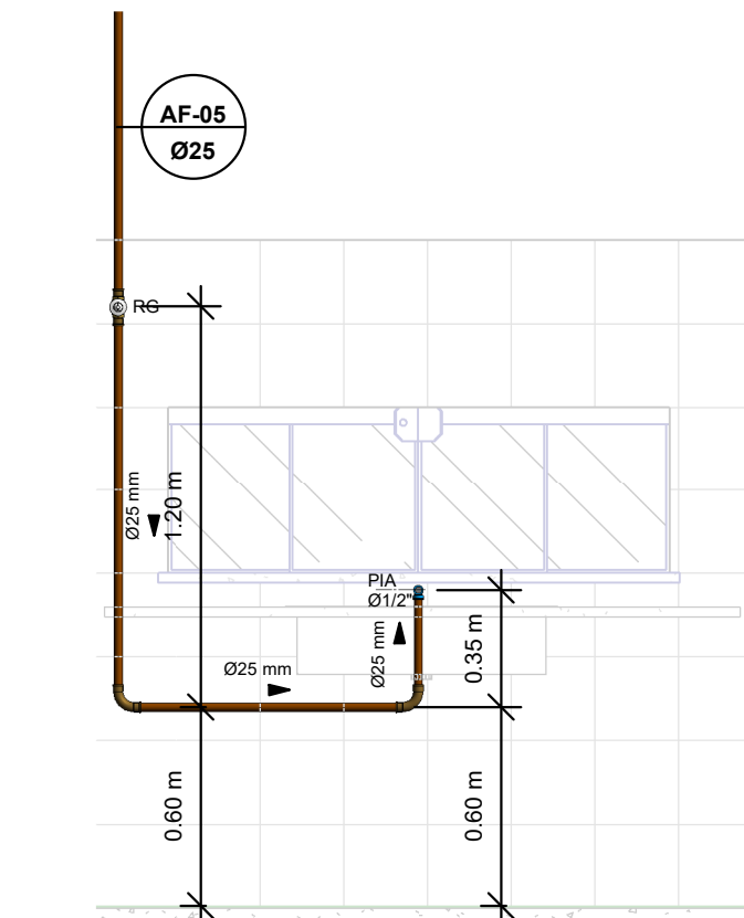
6 Elevação 04 1 : 25
