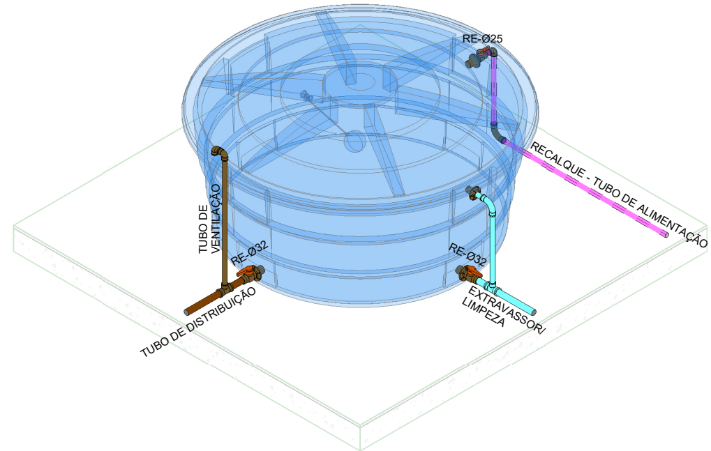
8 DETALHE -BARRILETE
