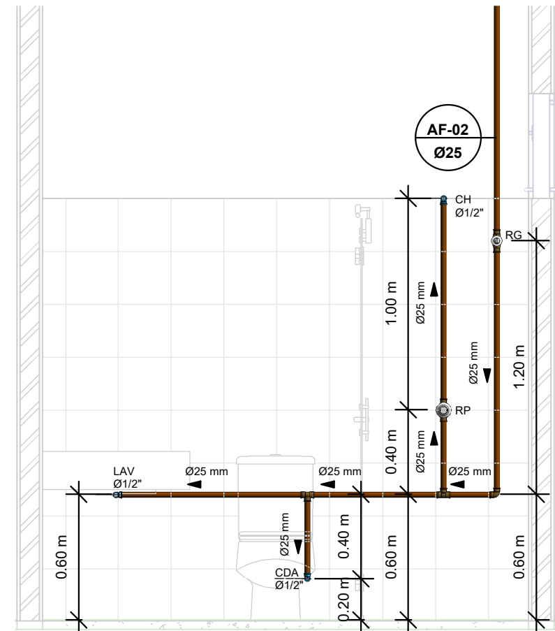
2 Elevação 01 1 : 25
