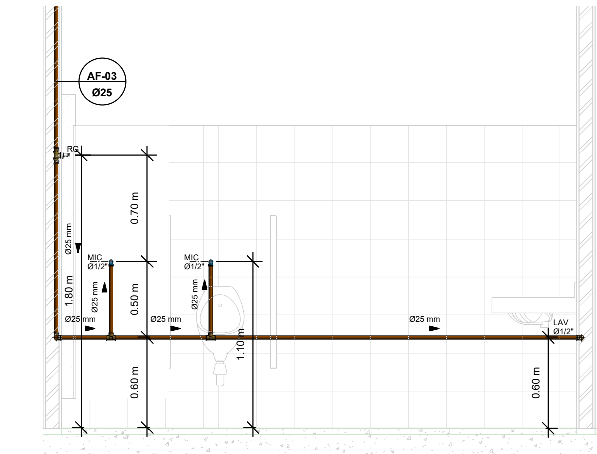
3 Elevação 02 1 : 25
