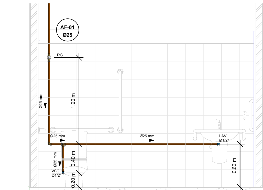
5 Elevação 03 1 : 25
