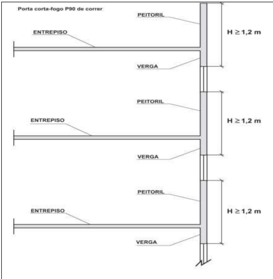
Figura A2 – Modelo de Compartimentação Vertical (verga-peitoril)
