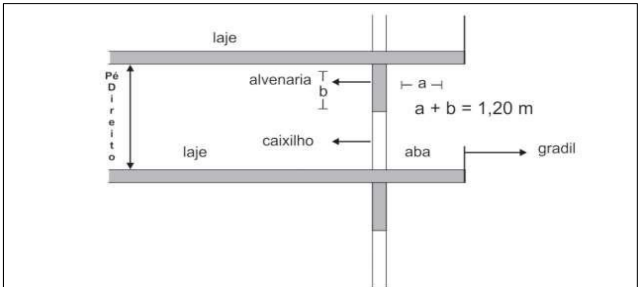
Figura A5 – Modelo de compartimentação vertical (composição entre aba e verga-peitoril)
