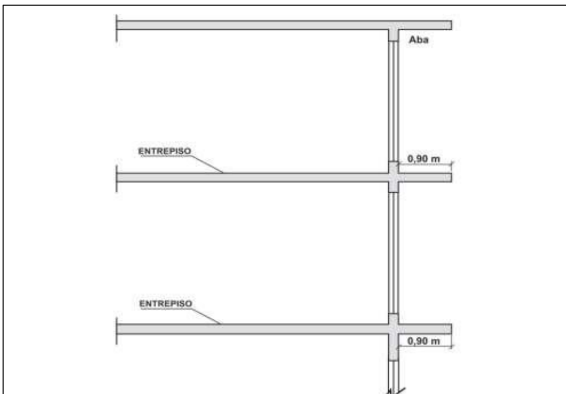
Figura A3 – Modelo de compartimentação vertical (abas)
