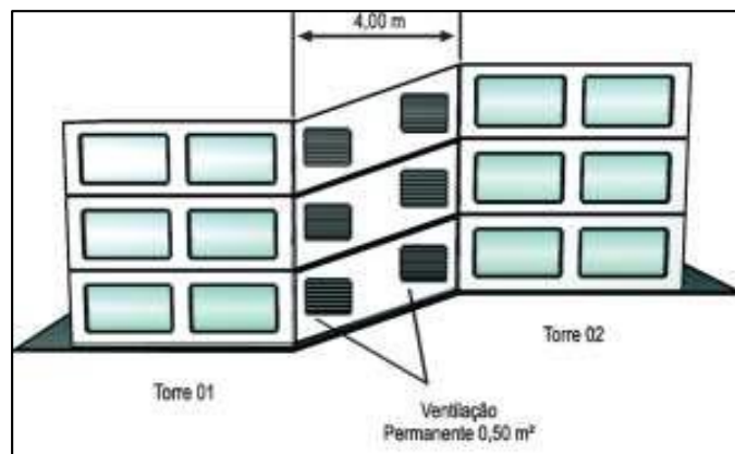
Figura 12 – Abertura lateral na escada
